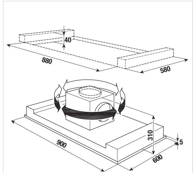
EDL 9750.1 E Paslanmaz çelik
