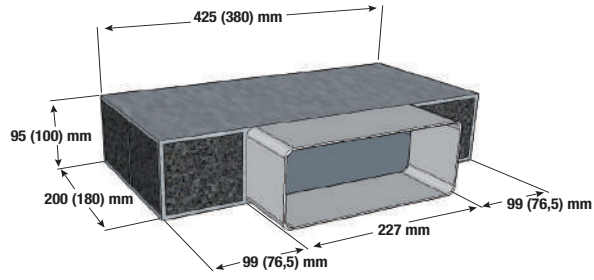
Karbon Filtre Kutusu ZK 8001 (ZKM 8051)
