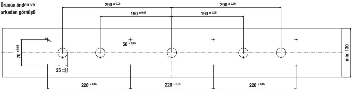
KMI 9850.0'ın Kontrol Paneli Kurulum Çizimleri
