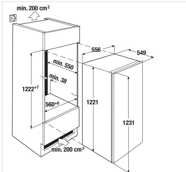
FK 4505.1i Mobilyaya sabitleme sistemi ile
