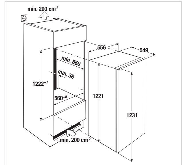
FK 4500.1i Mobilyaya sabitleme sistemi ile
