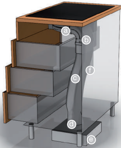
KURULUM ŞEMASI: EGZOS BORUSU
